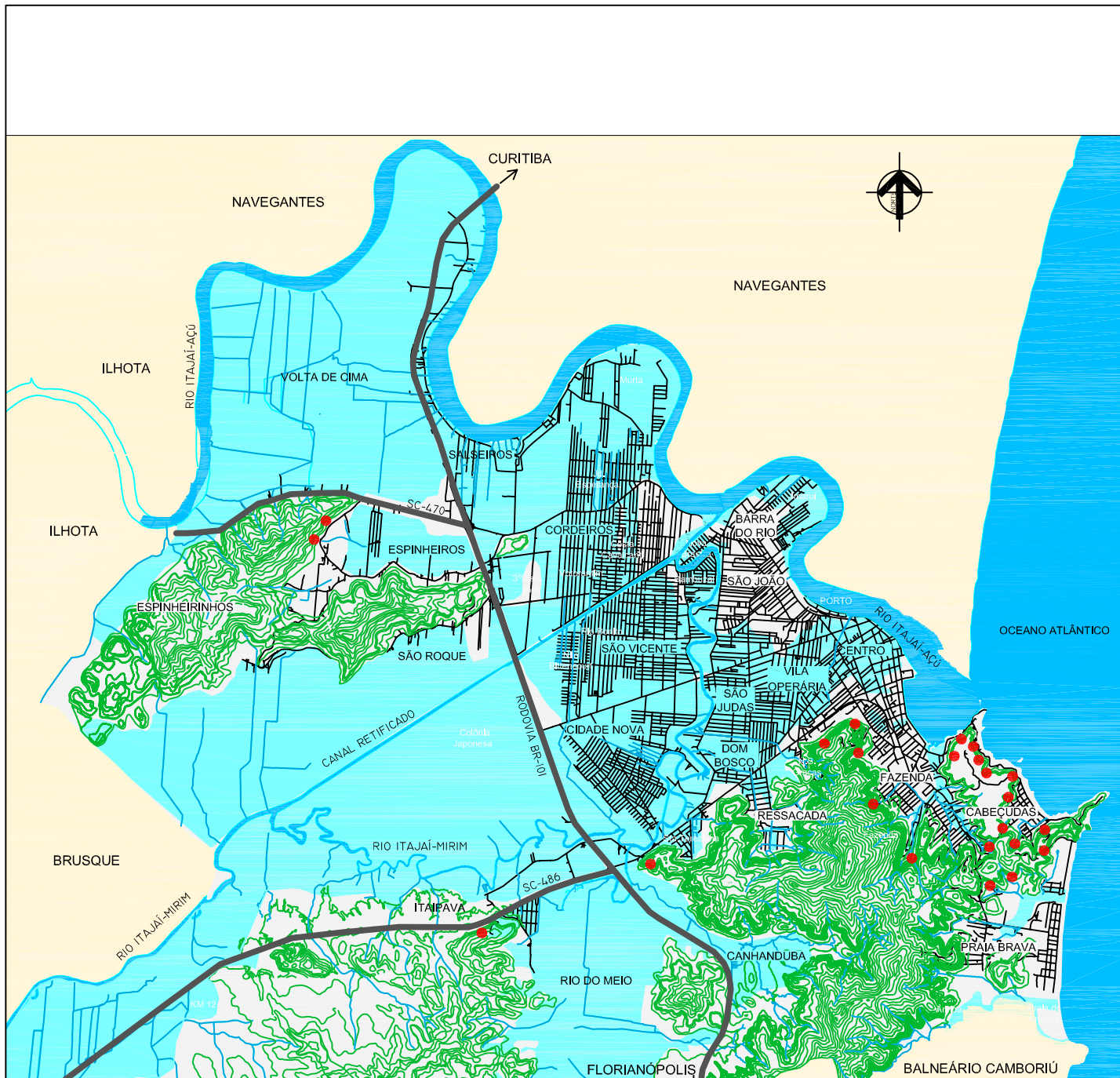
COTA DE ENCHENTE MAPEADA POR MODELO DIGITAL DE ELEVAÇÃO
